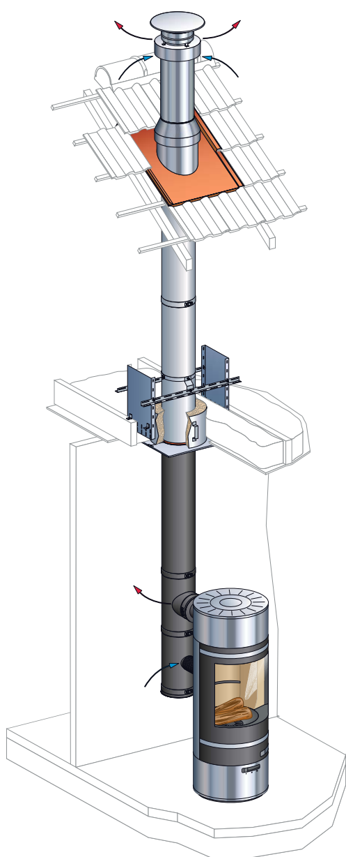
VNITŘNÍ KOMÍN S PŘÍVODEM VZDUCHU
