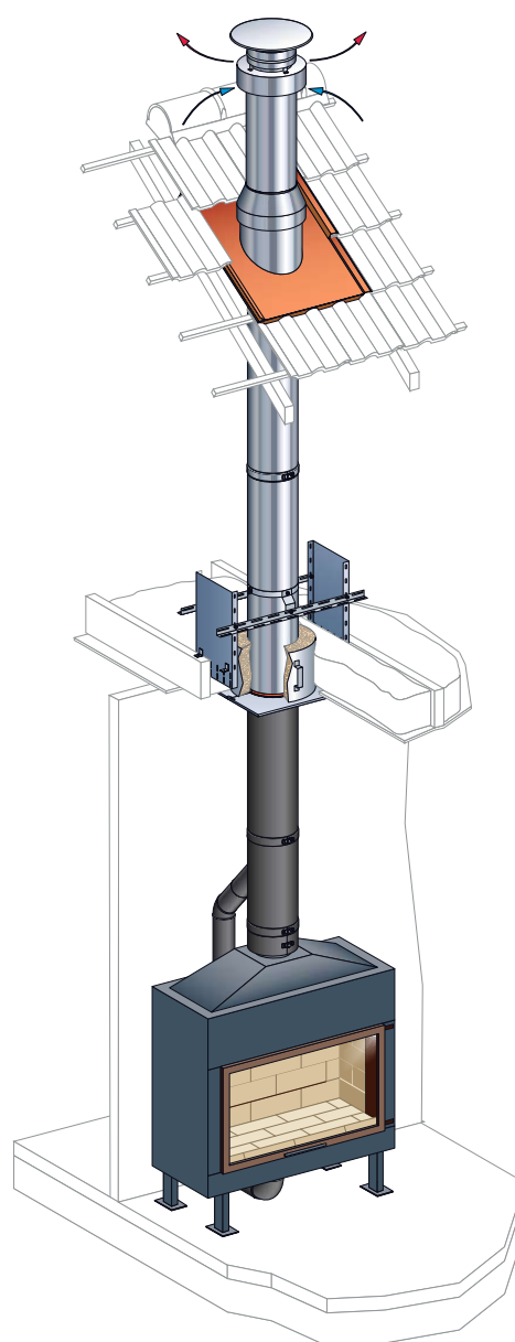
KOUŘOVOD S FUNKCÍ KOMÍNA S PŘÍVODEM VZDUCHU
