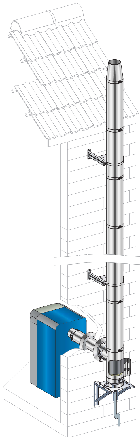
KOMÍN VNĚ BUDOVY
